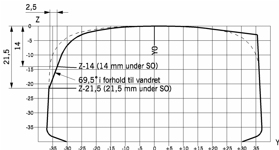
Figur 14.2-1 Illustration af skinneprofil NG5.
