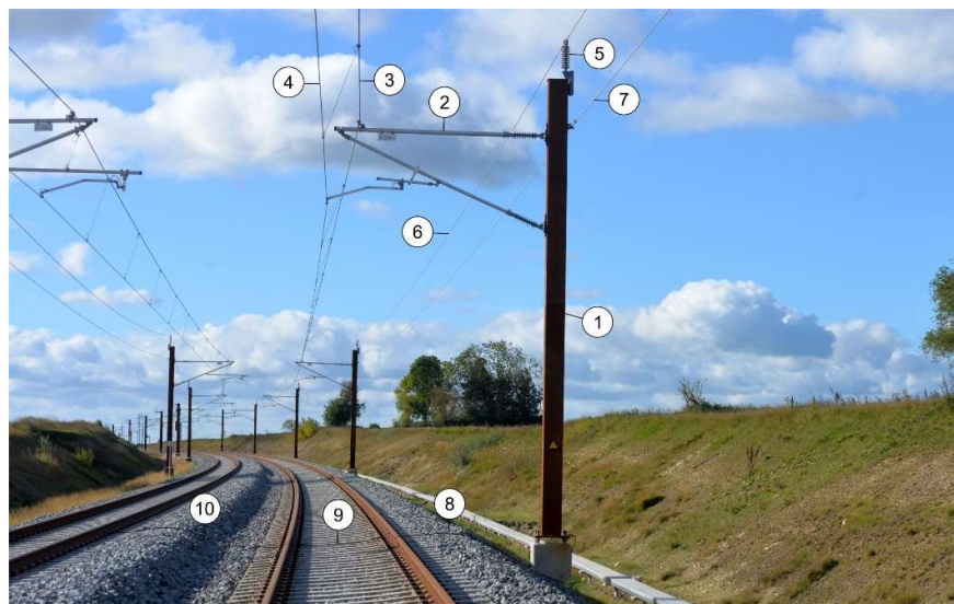
Figur Bilag 1.1–2 Eksempler på kørestrømsanlæggets komponenter
