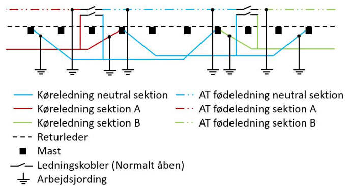
Figur 11.8.1-2 Arbejdsjording i "split" neutralsektion.
