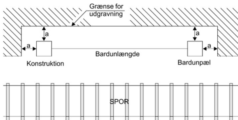
Figur 16.4-1: Grænse for opgravning nær fundament for køreledningskonstruktion med barduner.
