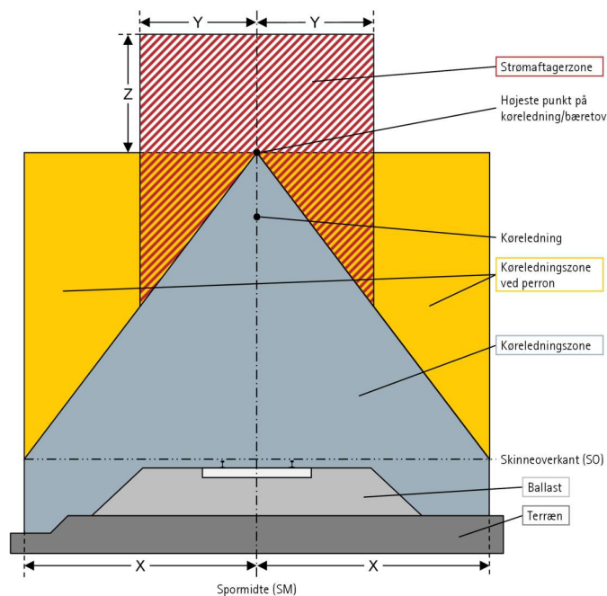
Figur 10.4.1-1 Profil af køreledningszonen og strømaftagerzonen.
