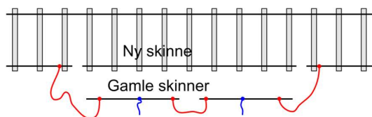
Figur 12.2.8.1-1 Rødmarkerede kabler er midlertidige kabelforbindelser (overstopninger), blåmarkerede kabler er returstrøms- eller potentialudligningsforbindelser.
