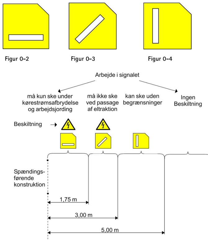
Figur 0-5 Betydning af beskiltning.
