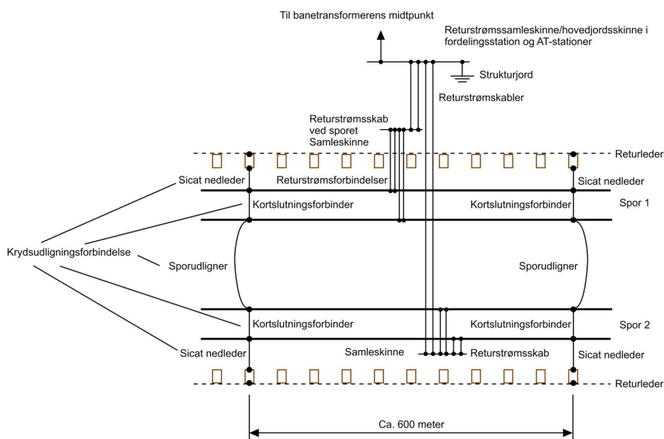
Figur Bilag 8.1-1 Principdiagram for returstrømsforbindelses-/kablernes tilslutningspunkter for et dobbeltspor.
