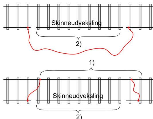
Figur 12.2.8.1-2 På stykket benævnt 1) må der ikke findes isolerende stød. På stykket benævnt 2) må der ikke findes returstrøms- eller potentialudligningsforbindelser. Rødmarkerede kabler er midlertidige kabelforbindelser (overstropninger).
